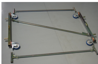
base di allargamento smontata
