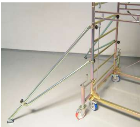
stabilizzatore ad aggancio rapido
