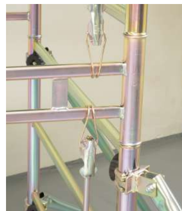
fissaggio delle crociere
